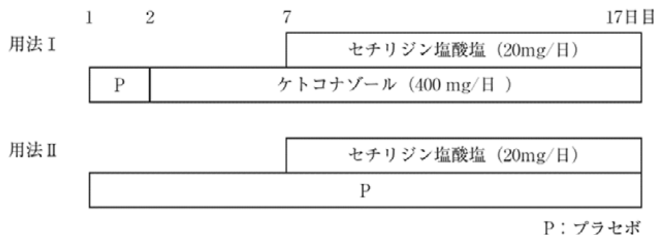
セチリジン塩酸塩（20mg/日）とケトコナゾール（400mg/日）の薬物動態学的相互作用
