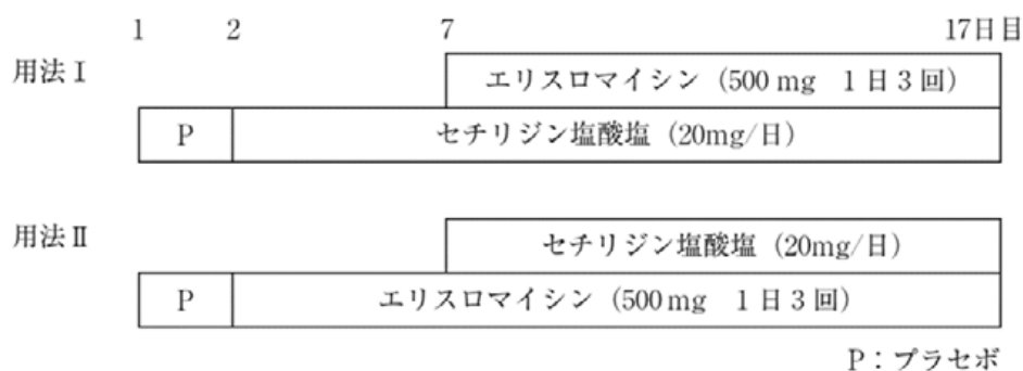
セチリジン塩酸塩（20mg/日）とエリスロマイシン（500mg×3/日）の薬物動態学的相互作用
